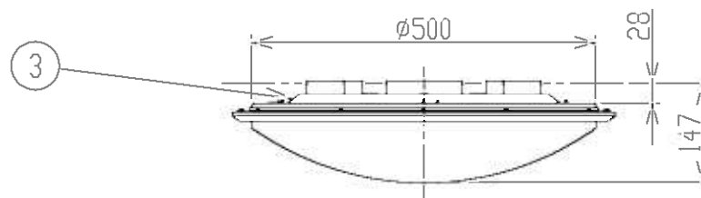
矢視 ②
