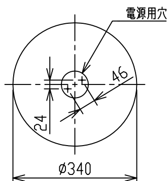
取付寸法(矢視 ㊸)
