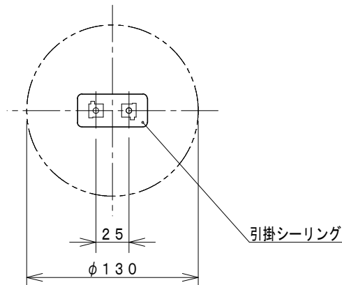
取付寸法 (矢視 a) (縮尺 1/4)
