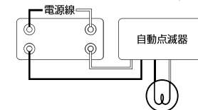
結線図
