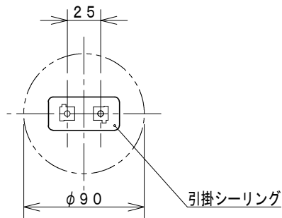
取付寸法（矢視 a） （縮尺 1/4）
