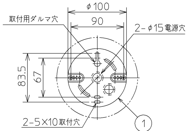
取付寸法（矢視α）
