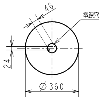
取付寸法（矢視 ㊦）
