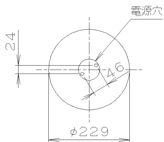
取付寸法（矢視a）
