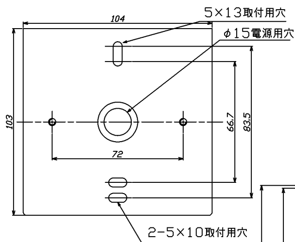
取付寸法 (矢視⑥)
