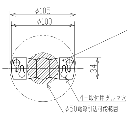
取付寸法(矢視a) (縮尺1/3)
