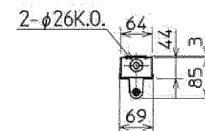
ボルト出ししろ
