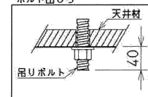
ボルト出ししろ
