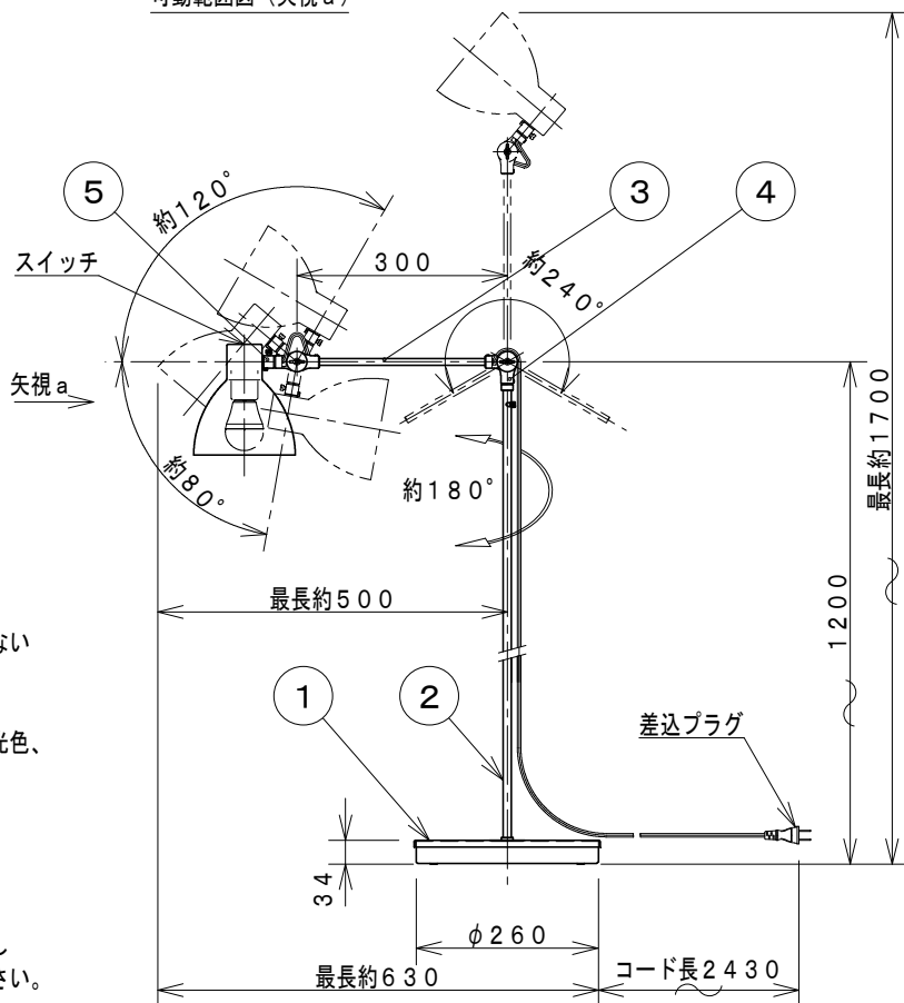
可動範囲図 (矢視 a)
