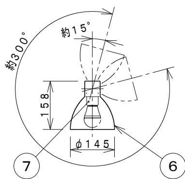
可動範囲図 (矢視 a)
