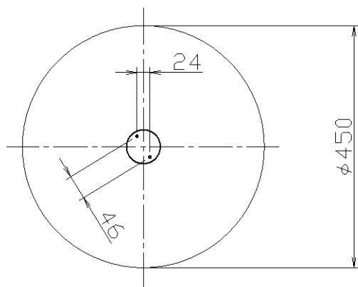
取付寸法（矢視 ①）
