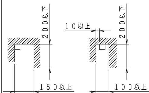
灯具最小施工寸法
