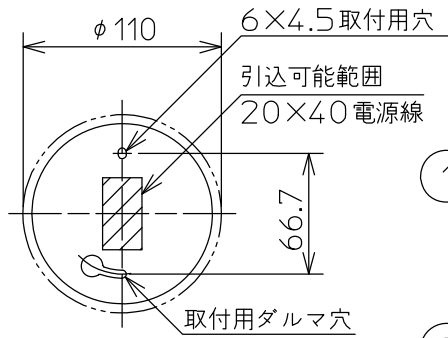
取付寸法 矢視a
