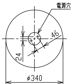
取付寸法(矢視 ②)
