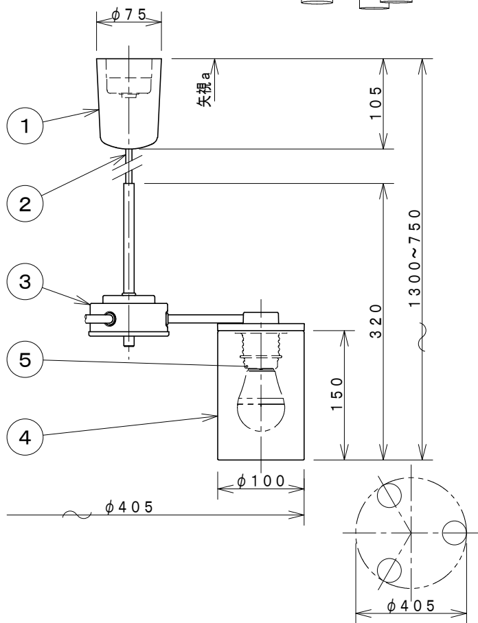
灯具配置図
