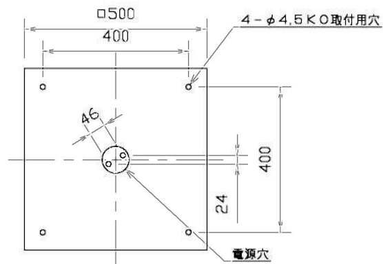
取付寸法 (矢視 ㊦)
