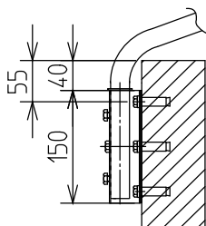
取付方向B図詳細図
