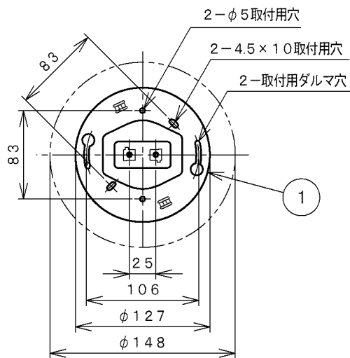
取付寸法（矢視 a）
