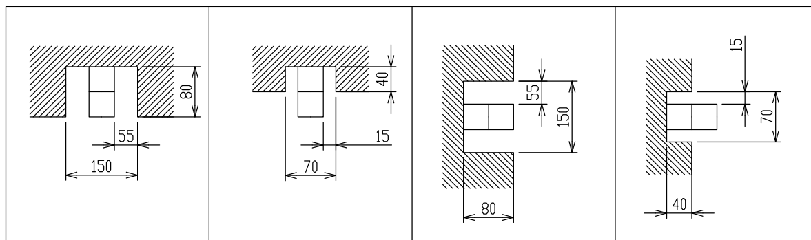
〈直付の場合〉
