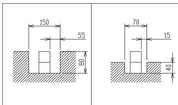
〈床置の場合〉
