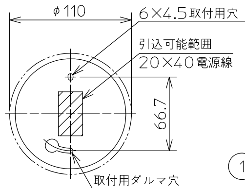
取付寸法 矢視a
