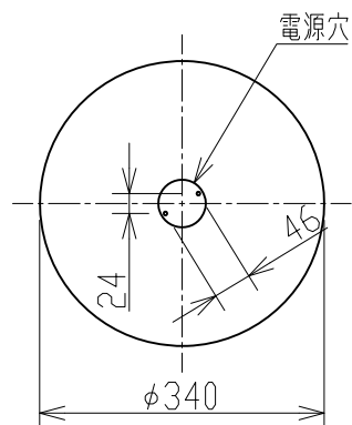
取付寸法(矢視a) (縮尺1/10)
