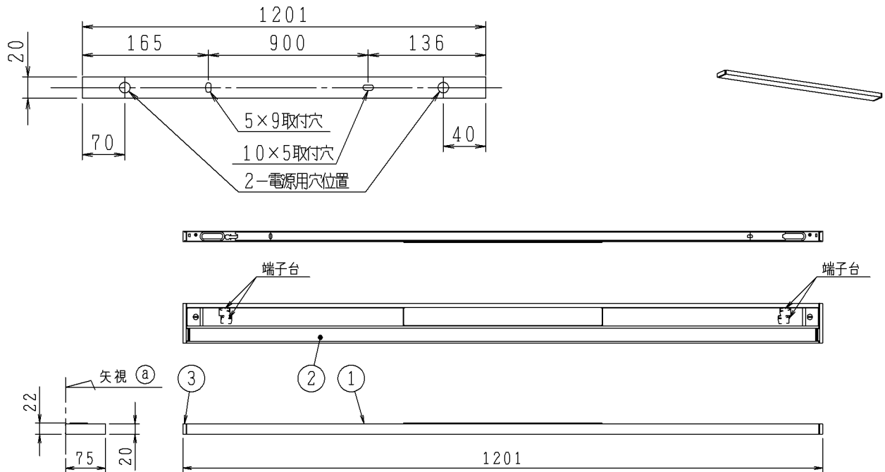
取付寸法（矢視 ㉔）
