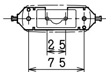
取付寸法(矢視⑧)
