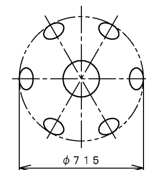
灯具配置図
