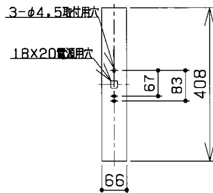
取付寸法 (矢視 ⑧)
