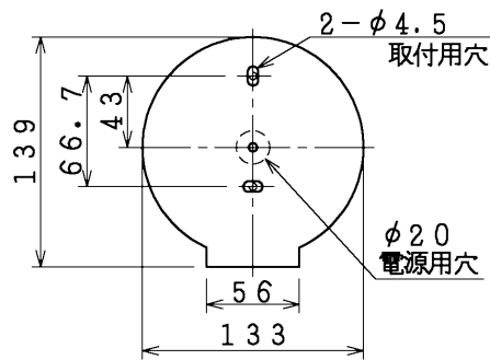
取付寸法 (矢視 ⑧)
