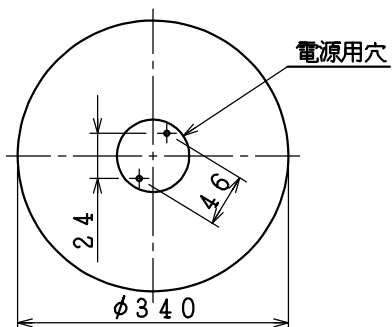
取付寸法(矢視 a)
