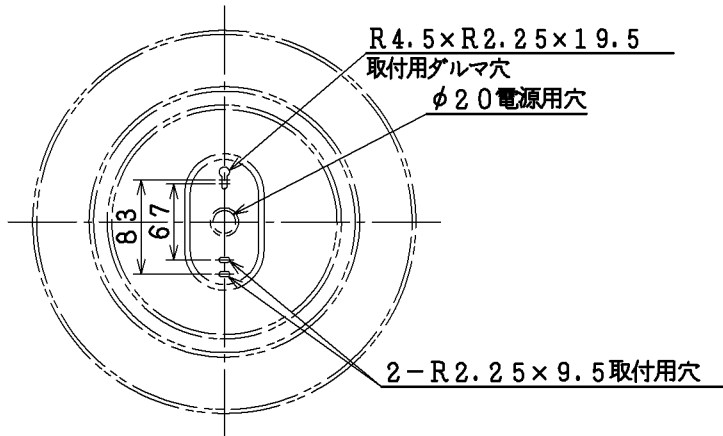
取付寸法(矢視①)
