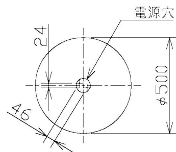
取付寸法（矢視㊸）
