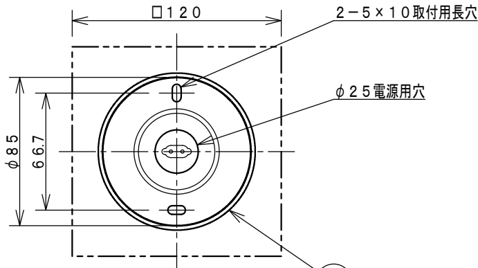
取付寸法 (矢視 a) (縮尺 1/3)
