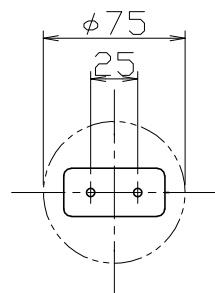
取付寸法（矢視 ㉔）
