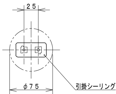
取付寸法 (矢視 a) (縮尺 1/4)
