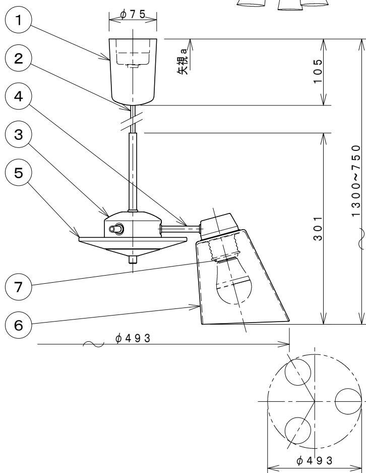
灯具配置図
