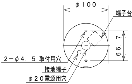
取付寸法(矢視①)
