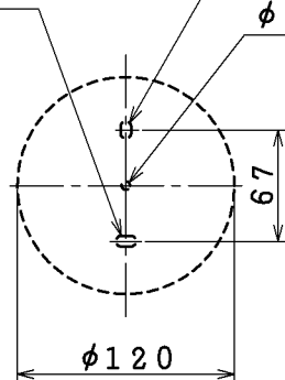
取付寸法（矢視 ⑧）
