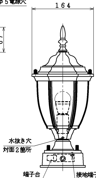
取付寸法（矢視 ⑧）
