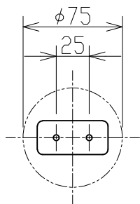
取付寸法(矢視a) (縮尺1/4)
