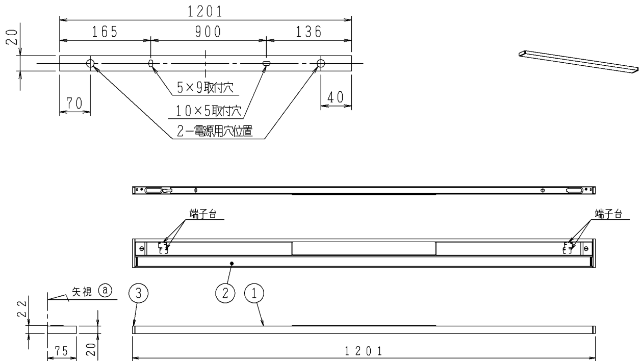
取付寸法（矢視 ㉔）
