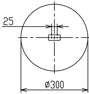
取付寸法(矢視 ④) (S=1/2)
