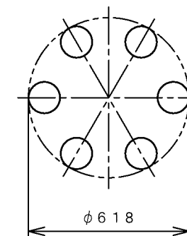
灯具配置図
