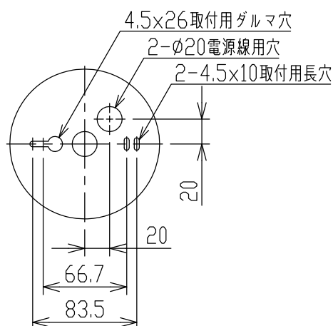
取付寸法(矢視 ②) S=1/2
