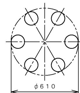
灯具配置図
