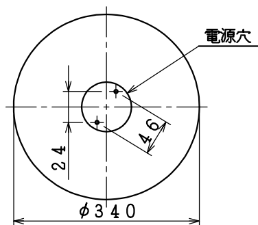
取付寸法 (矢視 a)
