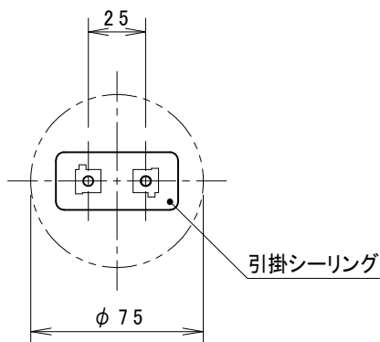
取付寸法(矢視a) (縮尺1/3)
