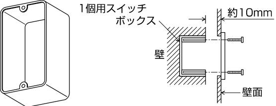
金属製スイッチボックス1個用(標準型またはカバー付) : JIS C 8340
