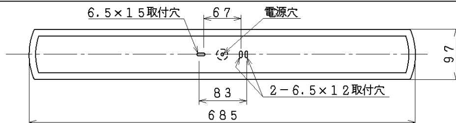
取付寸法（矢視 ②）
