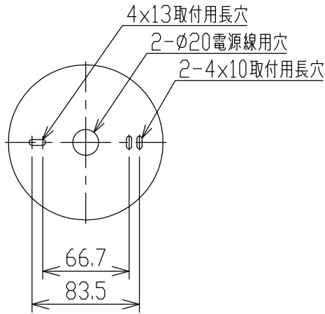
取付寸法(矢視 ①)
