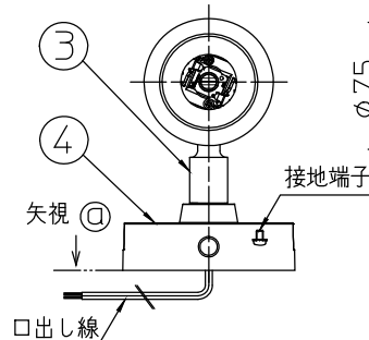
取付寸法(矢視 ㊟)
