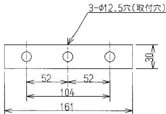
取付寸法〔矢視A〕
