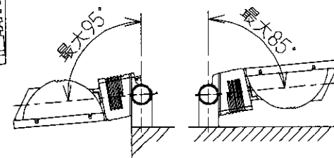
角度範囲説明図(例：クランド)
