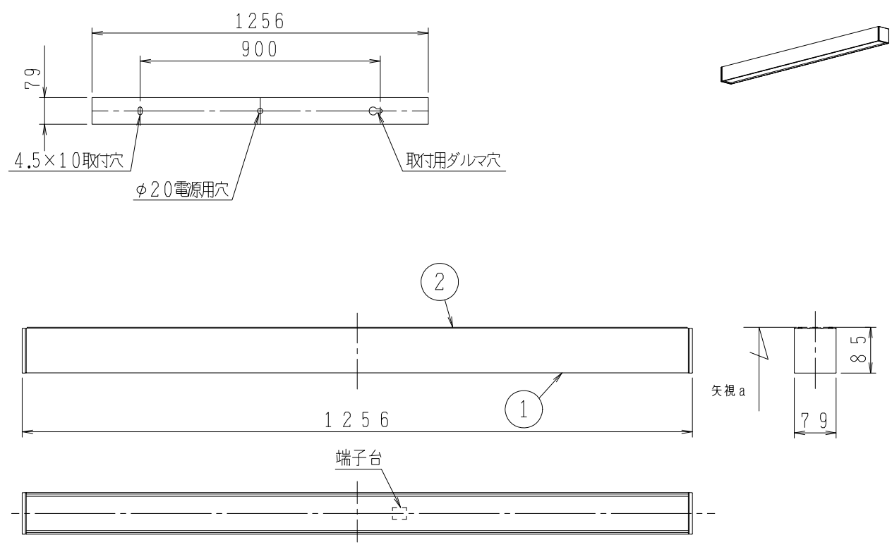
取付寸法（矢視 ㊸）
